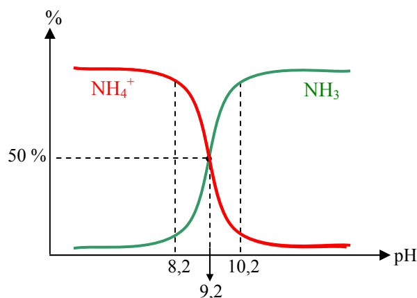
مخطط توزيع الصفة للثنائية \text{NH}_4^+ / \text{NH}_3
